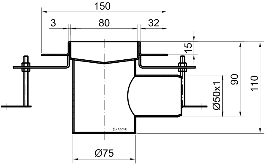
Schnitt A-A
