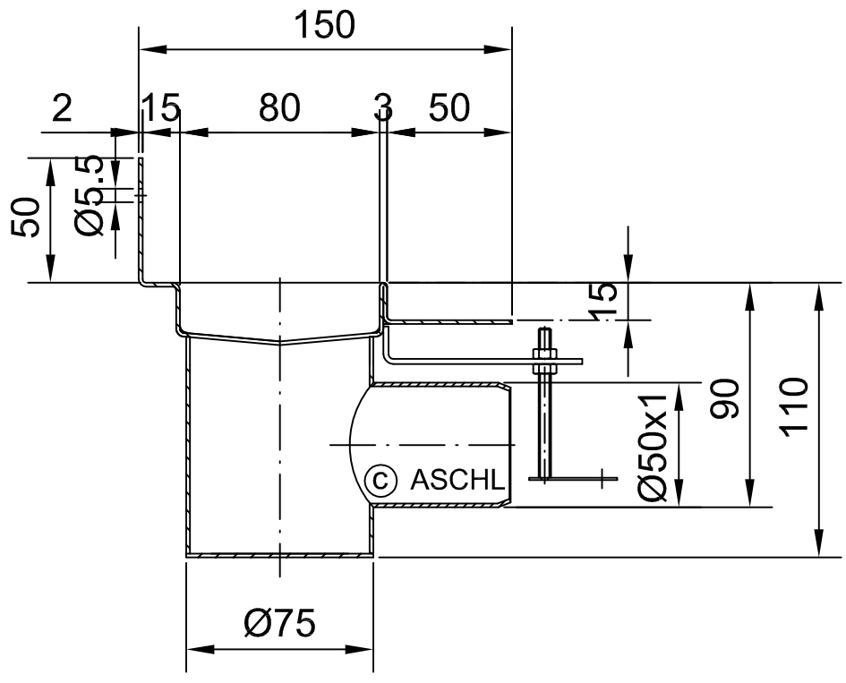
Schnitt A-A
