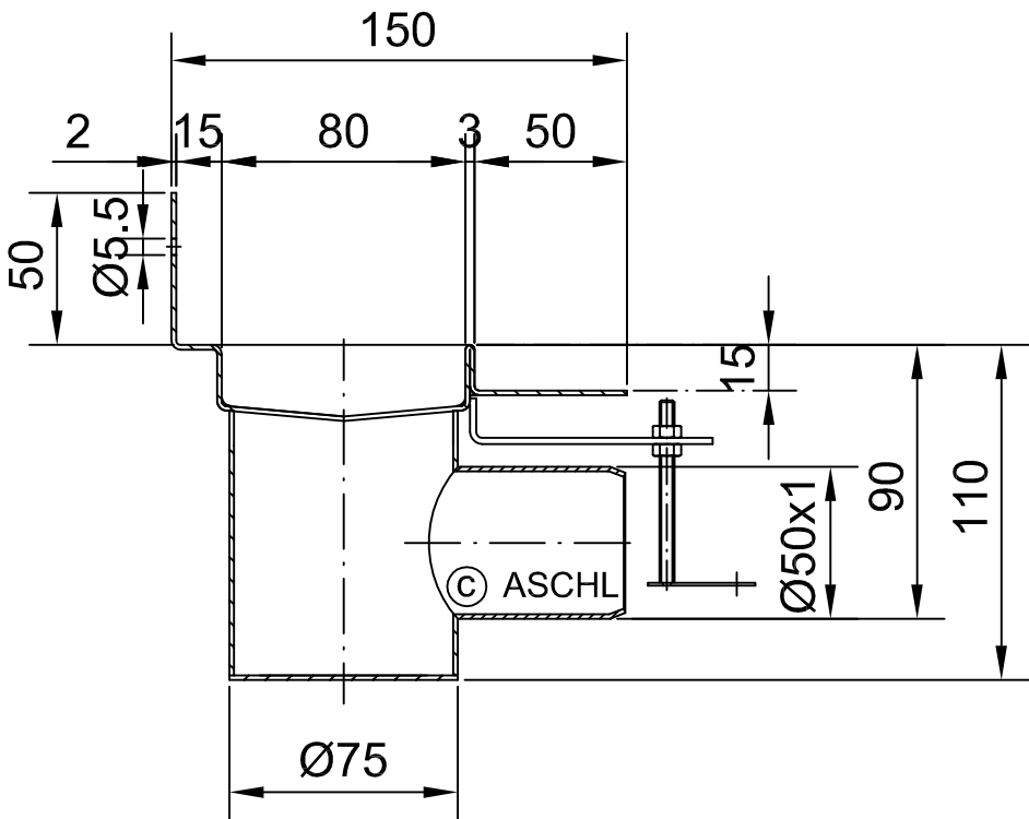
Schnitt A-A
