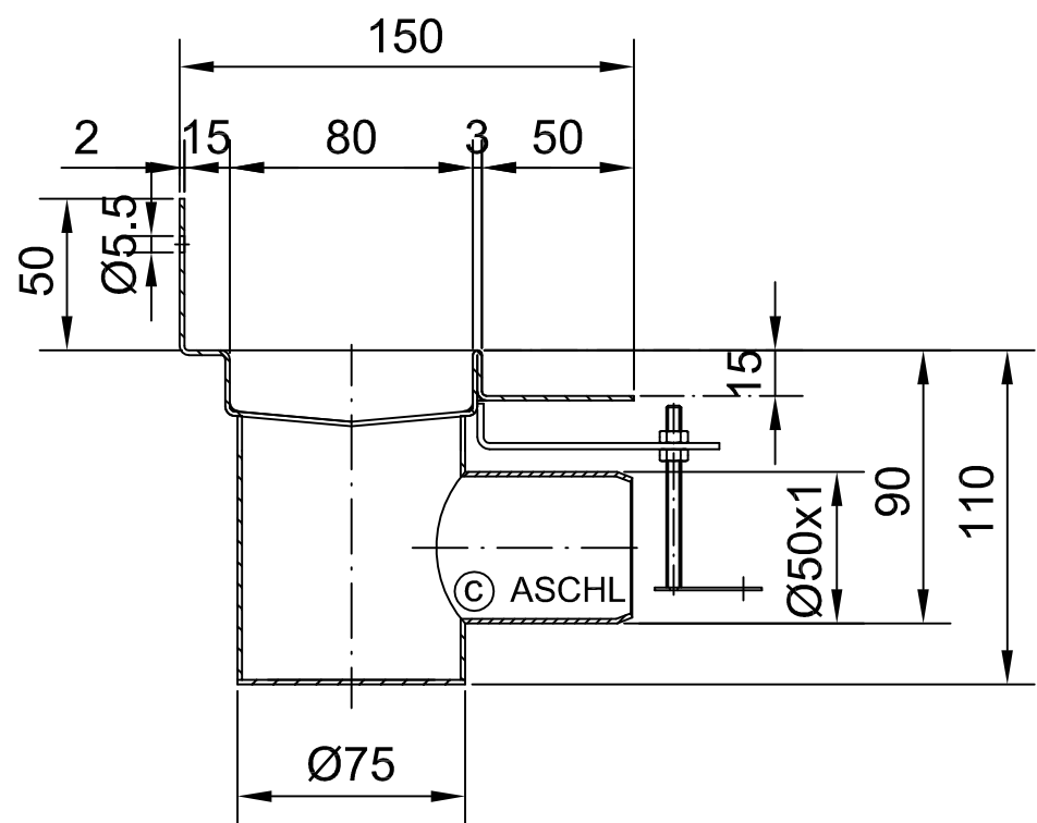
Schnitt A-A
