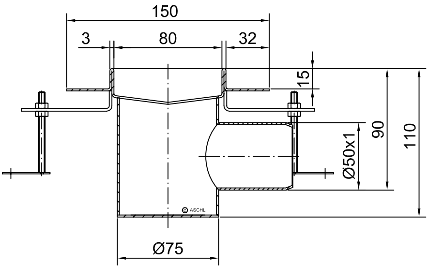
Schnitt A-A
