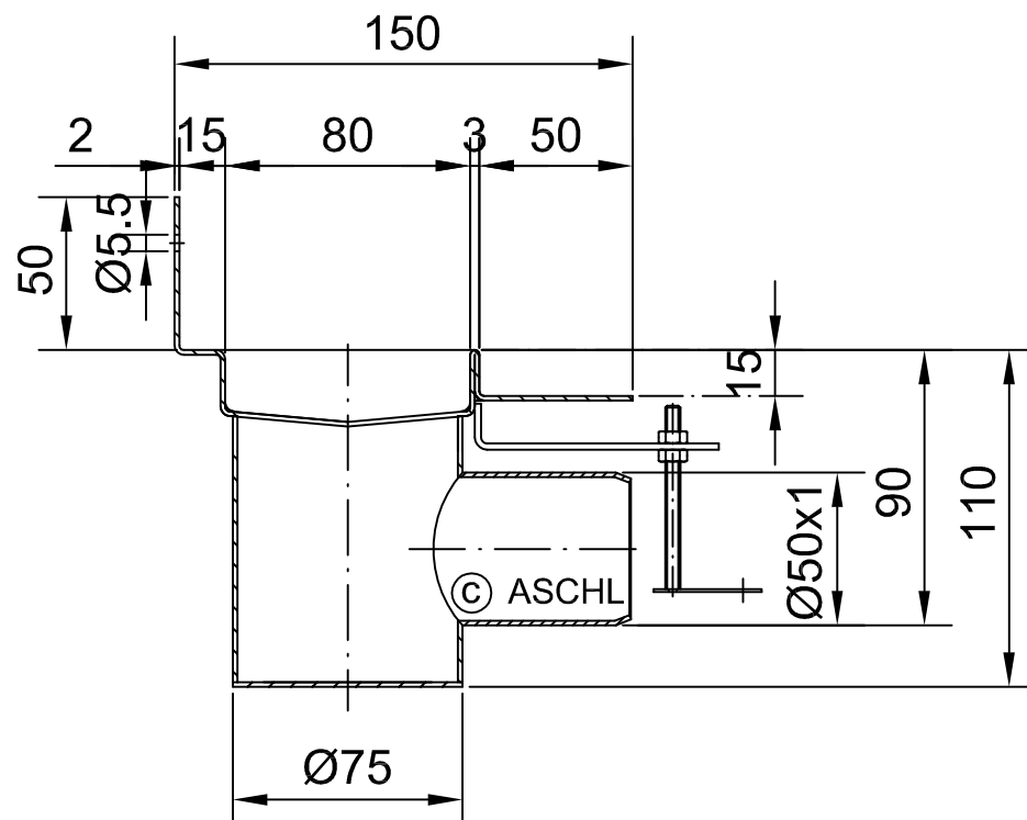
Schnitt A-A
